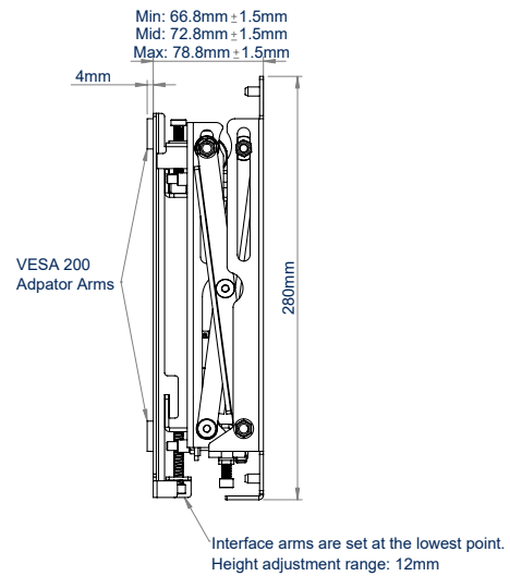
VISTA LATERAL CERRADO
