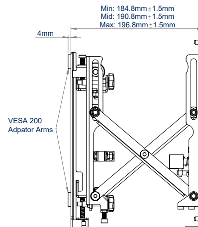
VISTA LATERAL AMPLIADO
