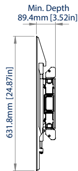
VISTA LATERAL A RAS DE LA PARED
