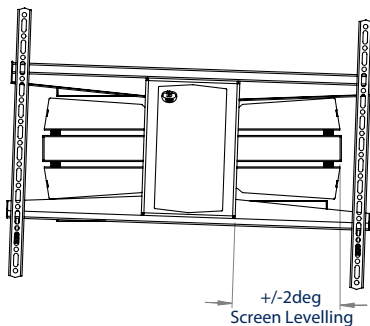
VISTA FRONTAL NIVELACIÓN DE LA PANTALLA
