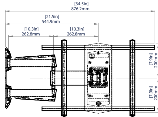
VISTA FRONTAL CON BRAZO EXTENDIDO HACIA UN LADO
