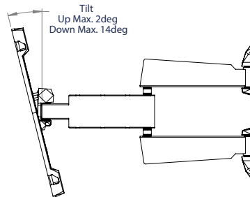
VISTA LATERAL EXTENSIÓN MÁXIMA
