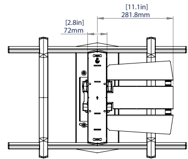
VISTA FRONTAL CON BRAZO EXTENDIDO HACIA UN LADO
