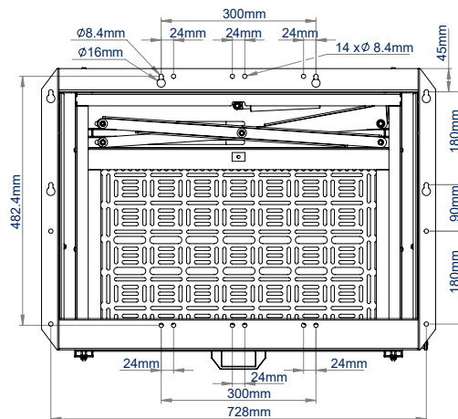
VISTA TRASERA
