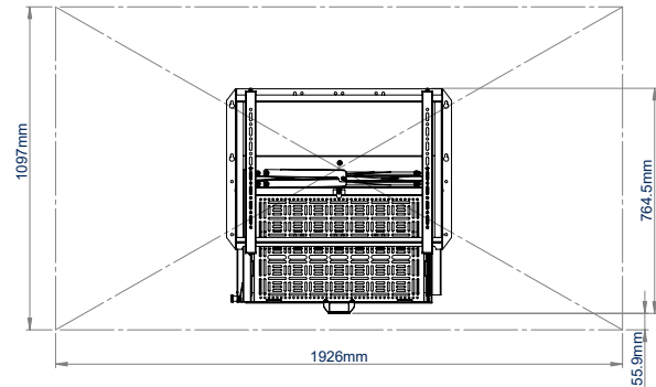
VISTA TRASERA 86" PANTALLA - CERRADA
