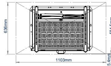
VISTA TRASERA 49" PANTALLA - CERRADA
