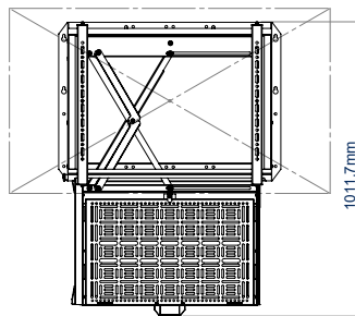
VISTA FRONTAL 49" PANTALLA - ABIERTA
