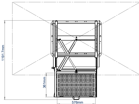
VISTA FRONTAL 86" PANTALLA - ABIERTA
