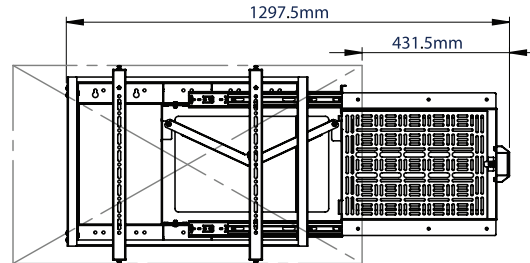
PANTALLA DE 46" ABRIR
