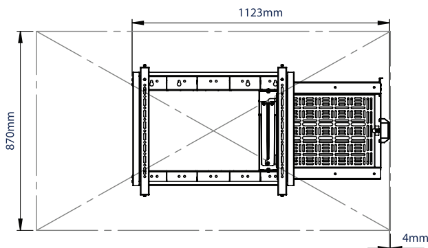
PANTALLA DE 75" CERRADA
