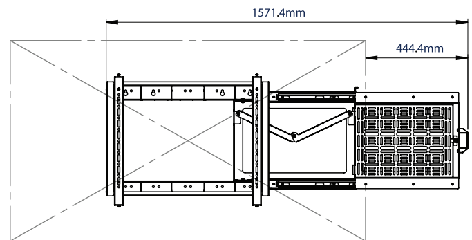
PANTALLA DE 75" ABRIR
