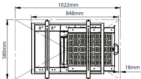
PANTALLA DE 46" CERRADO
