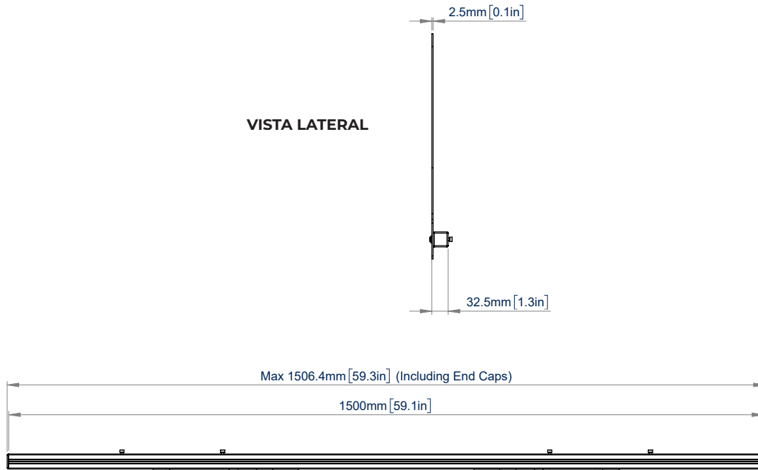
VISTA SUPERIOR
