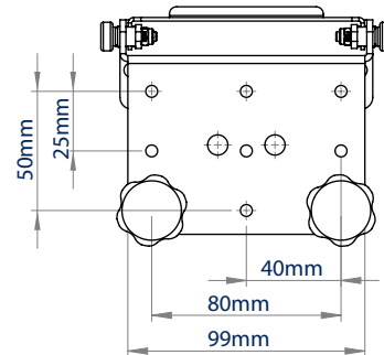
VISTA TRASERA
