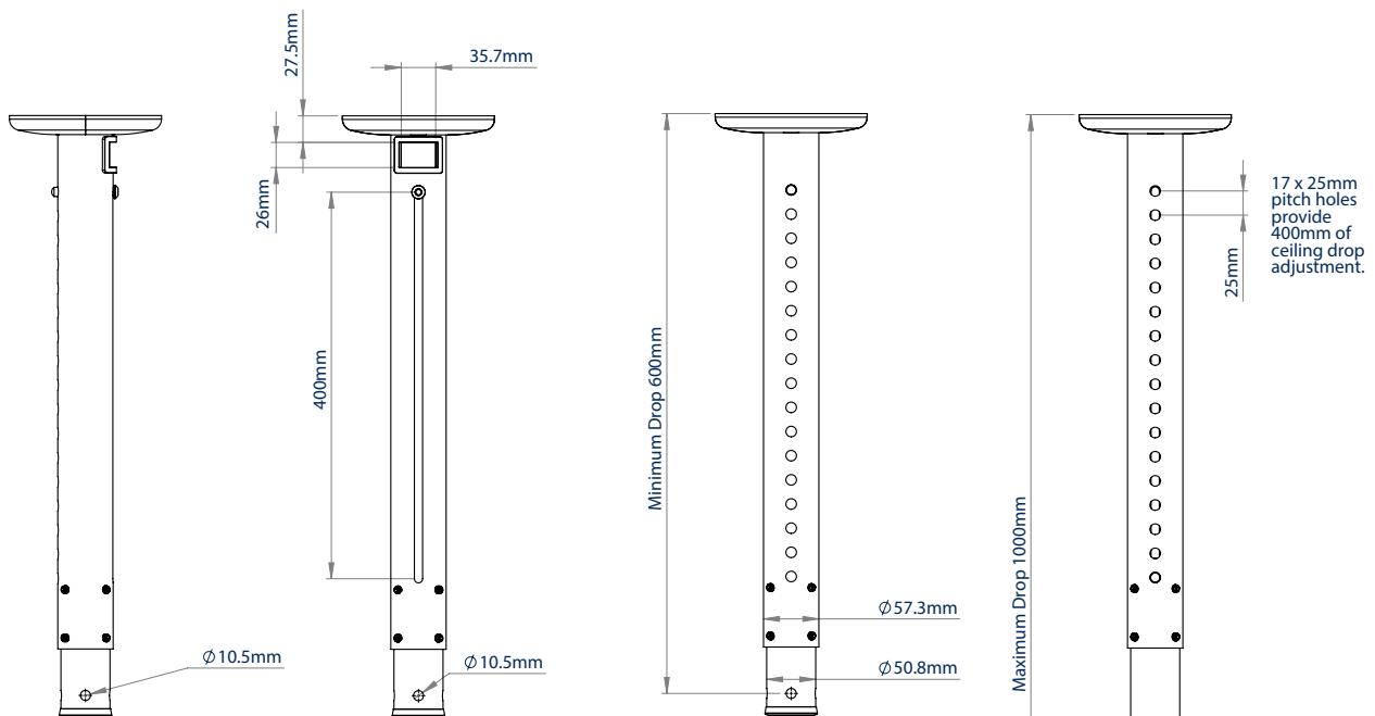
VISTA LATERAL
