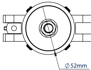
VISTA SUPERIOR
