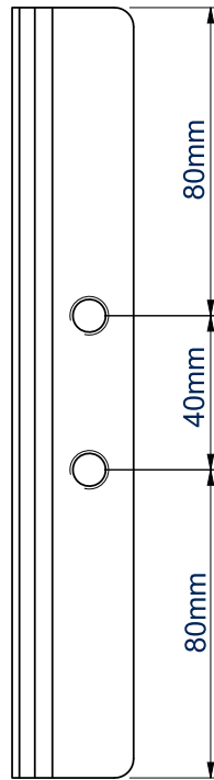
VISTA LATERAL
