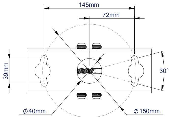
VISTA SUPERIOR
