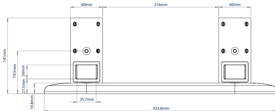
VISTA LATERAL CON PLACA DE CUBIERTA
