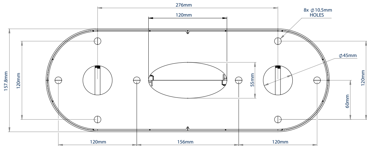
VISTA SUPERIOR CON PLACA DE CUBIERTA
