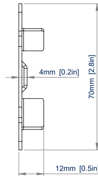
VISTA SUPERIOR
