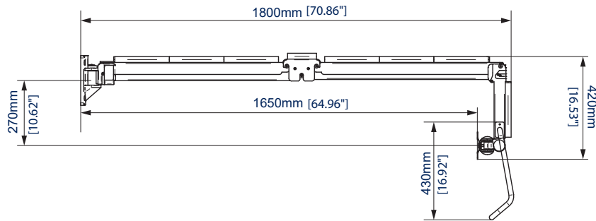
VISTA LATERAL EXTENSIÓN MÁXIMA
