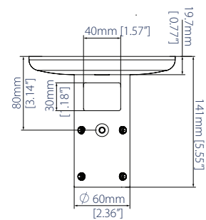
PLACA DE TECHO VISTA TRASERA
