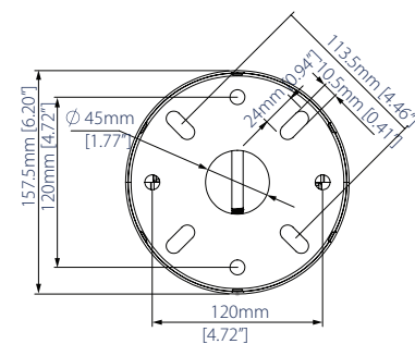
PLACA DE TECHO VISTA SUPERIOR
