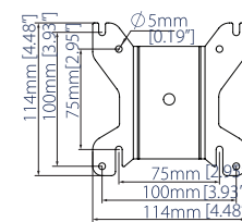
PLACA DE TECHO VISTA SUPERIOR
