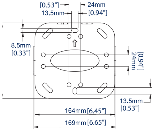
VISTA FRONTAL PLACA DE PARED
