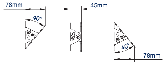
VISTA LATERAL SIN BRAZOS ADAPTADORES
