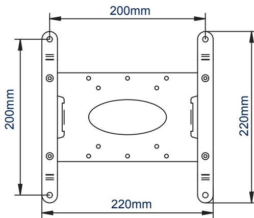
PLACA DE INTERFAZ CON BRAZOS ADAPTADORES VISTA FRONTAL
