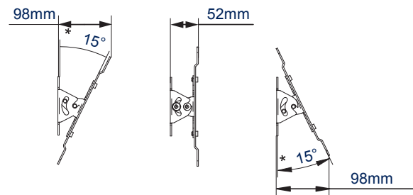
VISTA LATERAL CON BRAZOS ADAPTADORES
