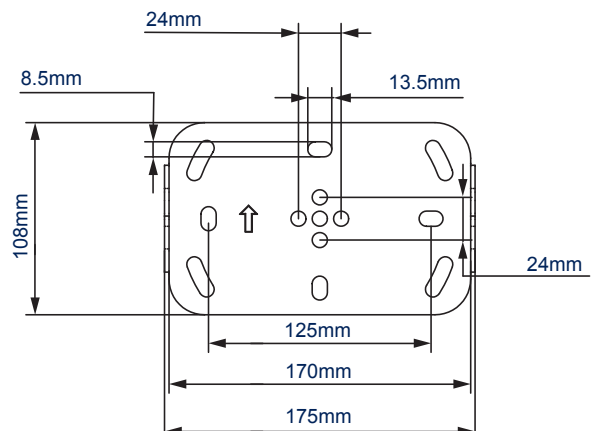
PLACA DE PARED VISTA FRONTAL
