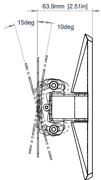
VISTA LATERAL
