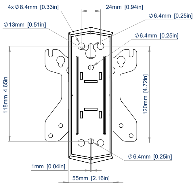
VISTA TRASERA
