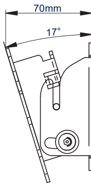
VISTA LATERAL INCLINADA HACIA ABAJO
