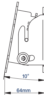
VISTA LATERAL INCLINADA HACIA ARRIBA
