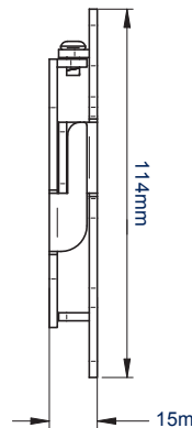
VISTA LATERAL PLACA DE PARED Y PLACA DE INTERFAZ
