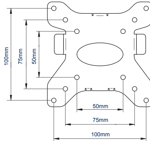
VISTA FRONTAL PLACA DE INTERFAZ
