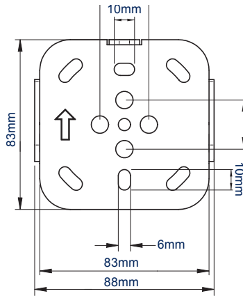
VISTA FRONTAL PLACA DE PARED
