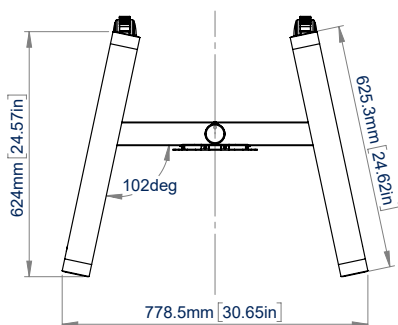
VISTA SUPERIOR
