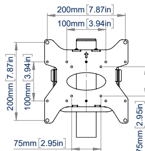
VISTA FRONTAL INTERFAZ PARA VESA FIJACIONES DE HASTA 200
