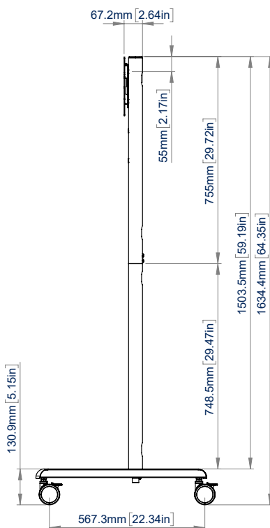
VISTA LATERAL
