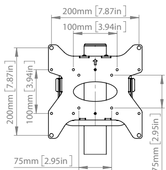
VUE AVANT INTERFACE POUR VESA JUSQU'À 200
