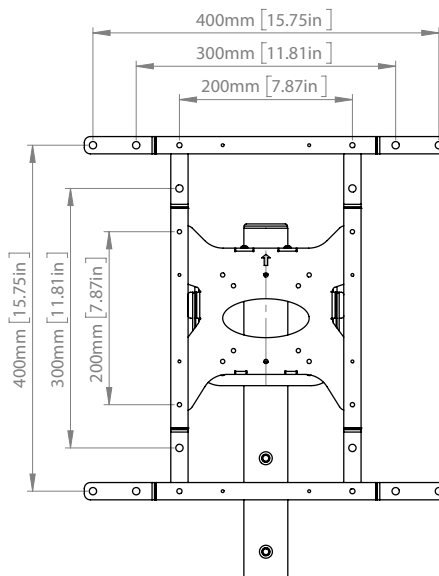
VUE AVANT INTERFACE POUR LES FIXATIONS VESA 400
