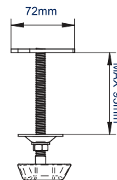
VISTA LATERAL OJAL
