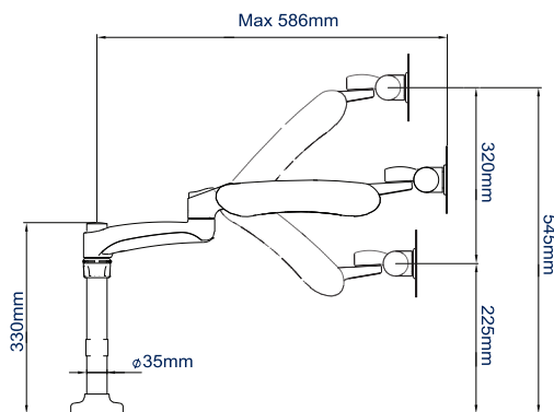
VISTA LATERAL
