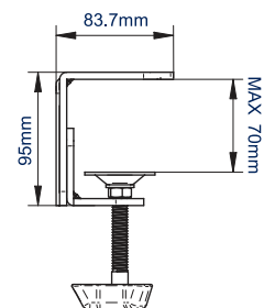
VISTA LATERAL ABRAZADERA DE MESA
