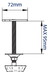
VISTA LATERAL GROMMET
