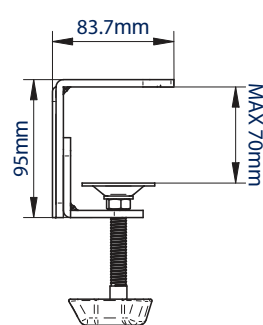
VISTA LATERAL ABRAZADERA DE MESA
