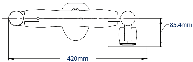
VISTA SUPERIOR
