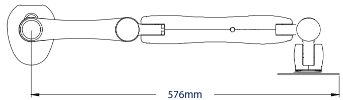
VISTA SUPERIOR EXTENSIÓN MÁXIMA
