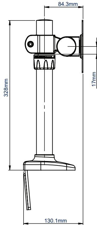
VISTA LATERAL
