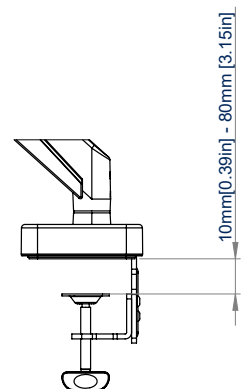
ABRAZADERA DE ESCRITORIO
