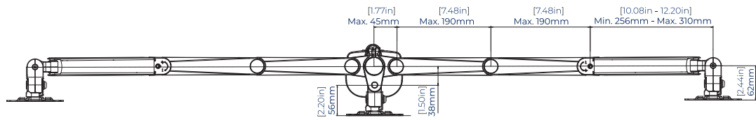
VISTA SUPERIOR
