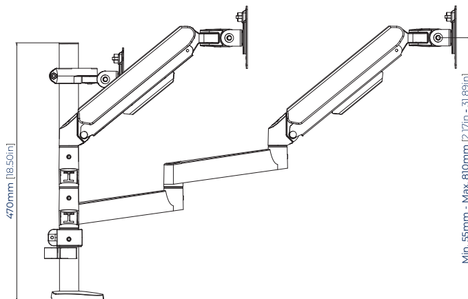
VISTA LATERAL
