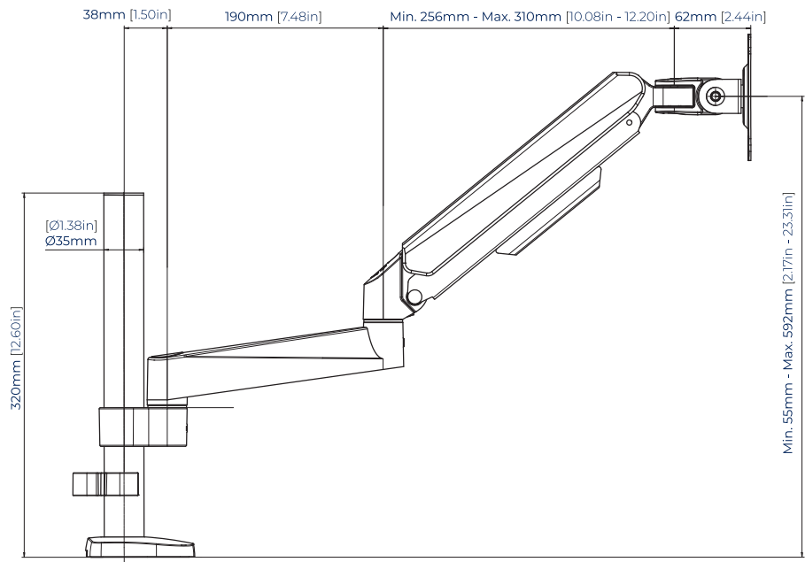
VISTA LATERAL
