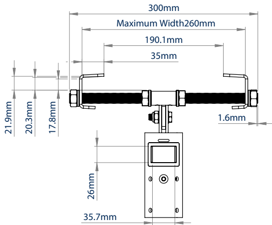
VISTA FRONTAL ANCHO MÁXIMO
