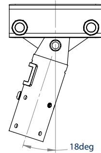
AJUSTE DE INCLINACIÓN 18 GRADOS
