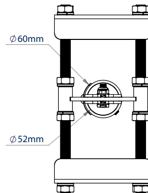
VISTA SUPERIOR
