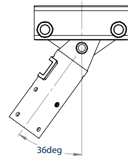
AJUSTE DE INCLINACIÓN 36 GRADOS (MÁXIMO)
