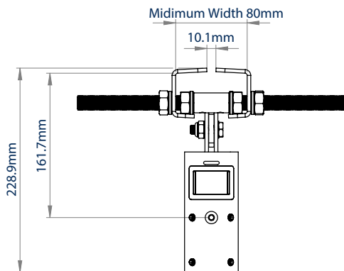
VISTA FRONTAL ANCHO MÍNIMO
