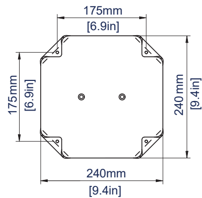
PLACA BASE
