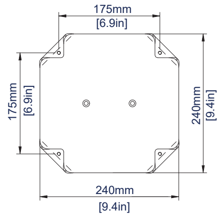
PLACA BASE
