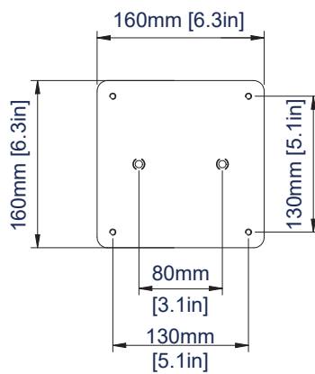
PLACA SUPERIOR
