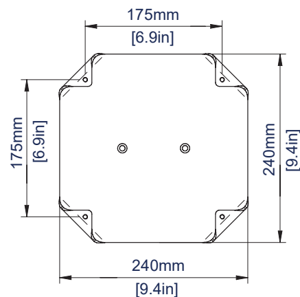
PLACA BASE
