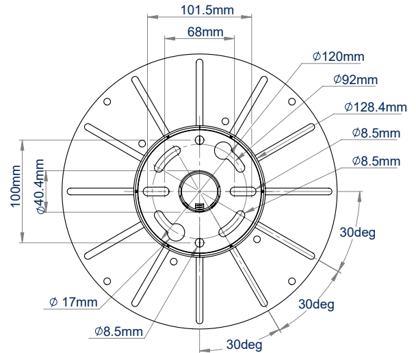
PLACA DE TECHO VISTA SUPERIOR
