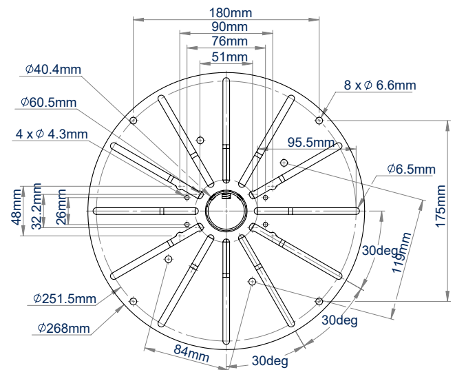
SOPORTE PARA CÁMARA DE CIRCUITO CERRADO VISTA INFERIOR
