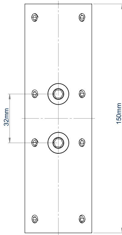
VISTA LATERAL
