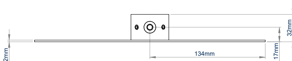
VISTA LATERAL
