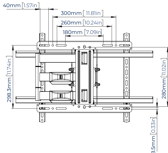
VISTA TRASERA
