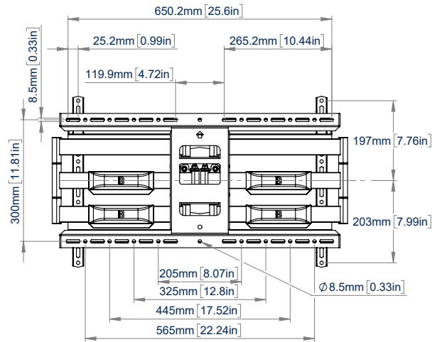
VISTA TRASERA
