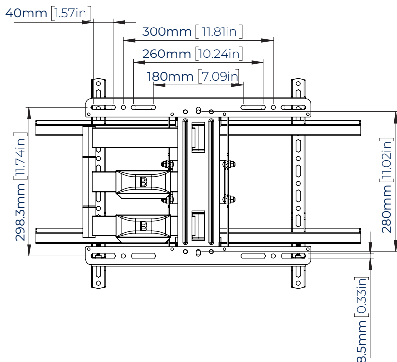
VISTA TRASERA
