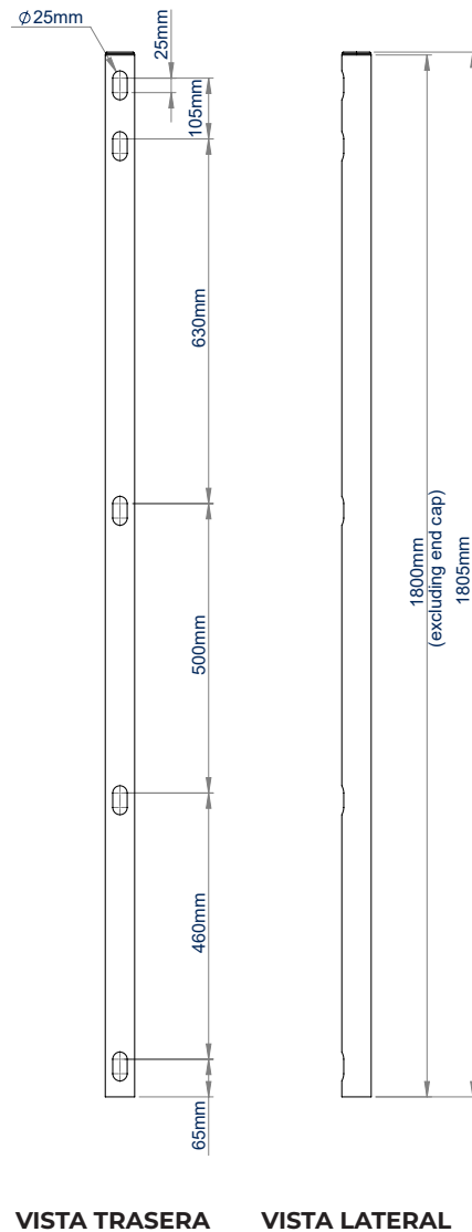
VISTA TRASERA
