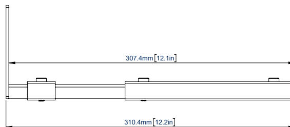
VISTA LATERAL
