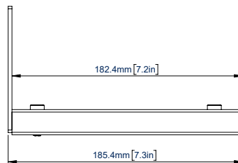
VOORAANZICHT
