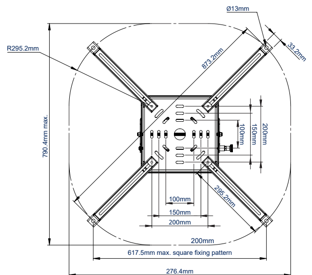
VUE DU DESSOUS AVEC GRANDS PIEDS EXTENSIBLES
