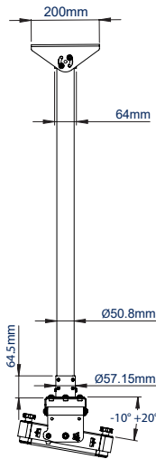
VUE LATÉRALE AFFICHAGE DE L'INCLINAISON
