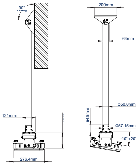
VUE LATÉRALE FIXATION MURALE
