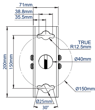
PLAQUE DE PLAFOND / MURALE
