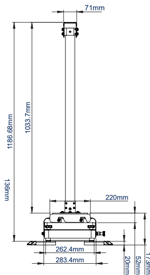
VUE DE FACE AVEC PIEDS D'EXTENSION
