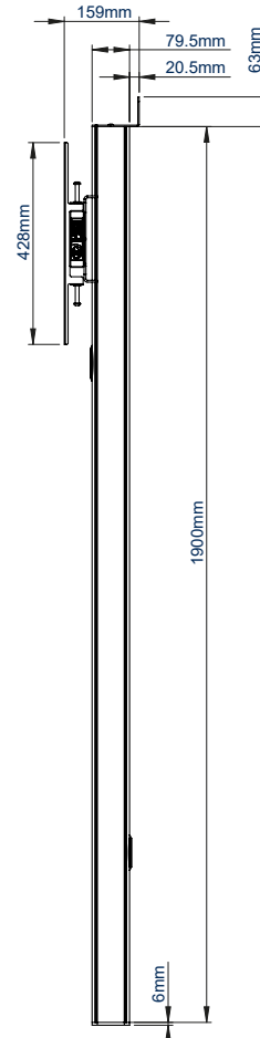
VUE LATÉRALE
