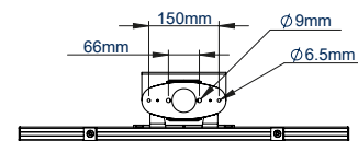
VUE ARRIÈRE
