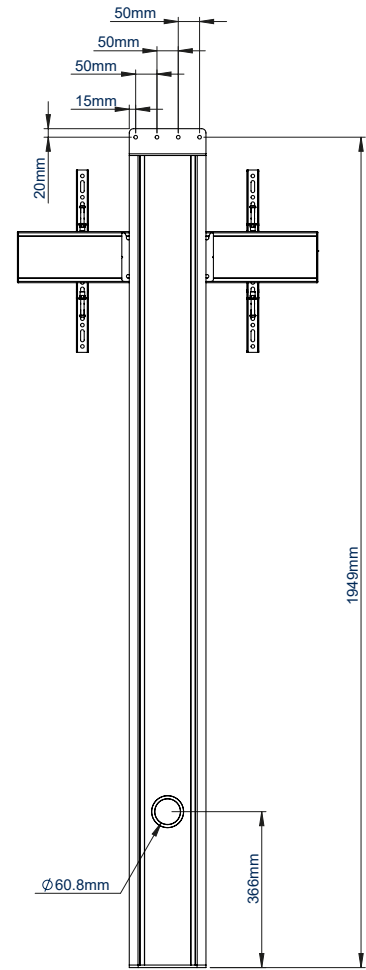
VUE ARRIÈRE
