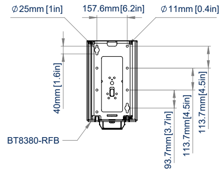
VUE DE DESSOUS BASE RÉTRACTABLE
