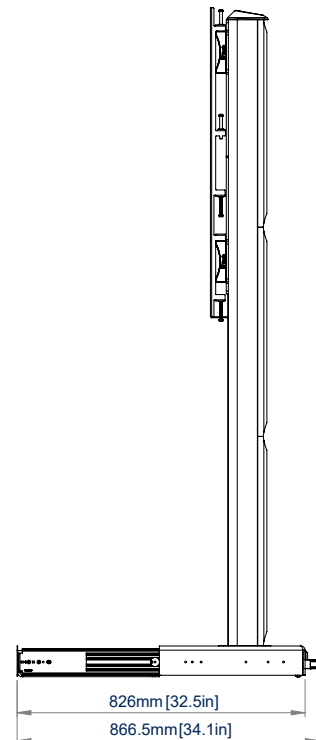
VUE LATÉRALE ÉTENDU
