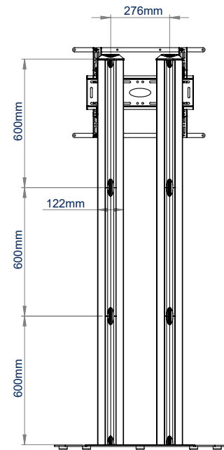
VUE ARRIÈRE
