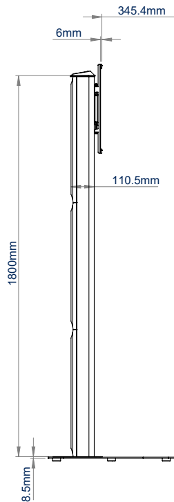
VUE LATÉRALE
