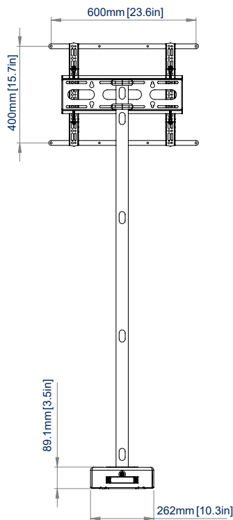
VUE ARRIÈRE
