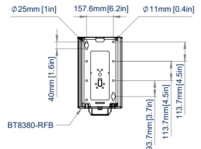
VUE DE DESSOUS BASE RÉTRACTABLE
