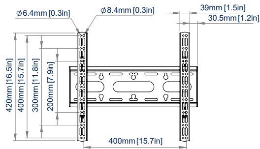
VUE DE FACE INTERFACE
