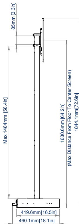
VUE LATÉRALE
