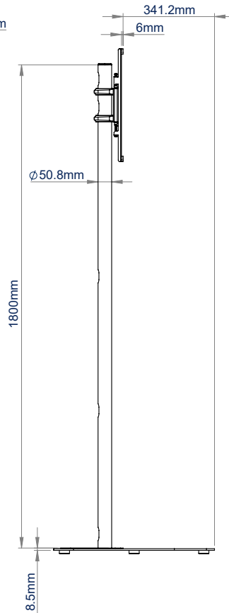
VUE LATÉRALE
