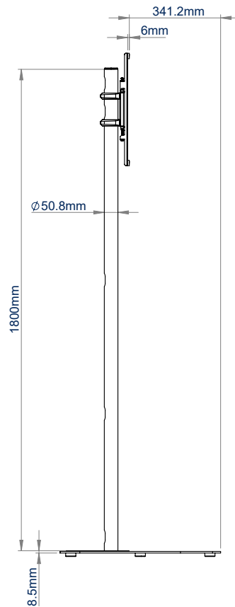
VUE LATÉRALE
