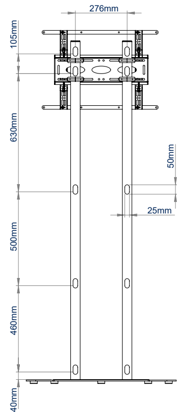
VUE ARRIÈRE
