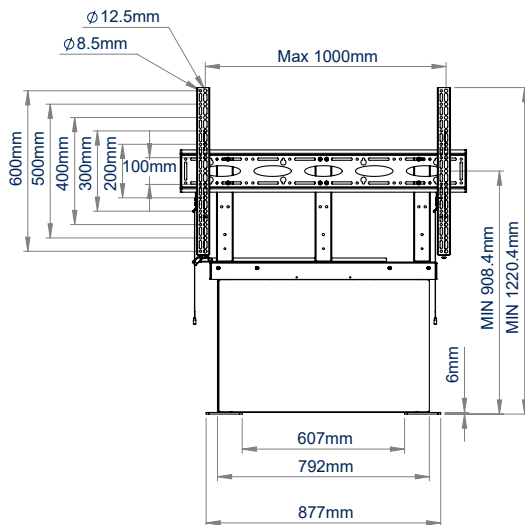
VUE ARRIÈRE POSITION LA PLUS BASSE
