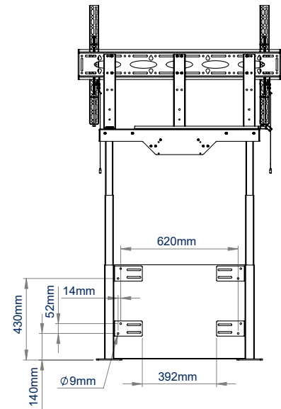
VUE ARRIÈRE POSITION LA PLUS ÉLEVÉE
