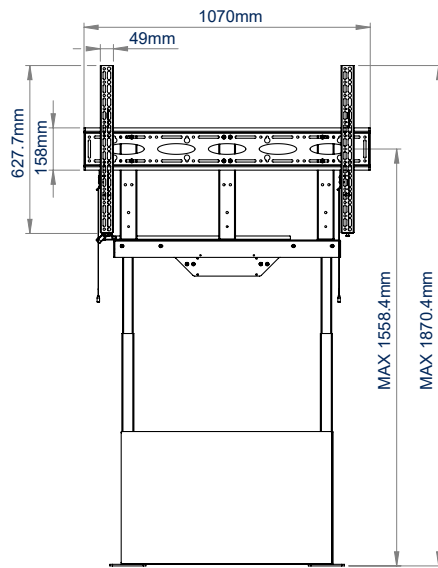
VUE DE FACE POSITION LA PLUS ÉLEVÉE
