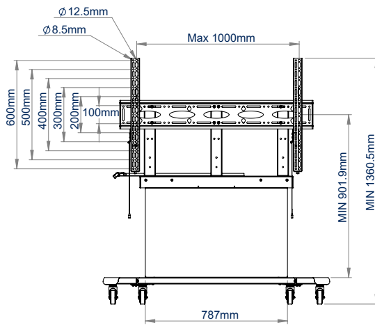
VUE ARRIÈRE POSITION LA PLUS BASSE
